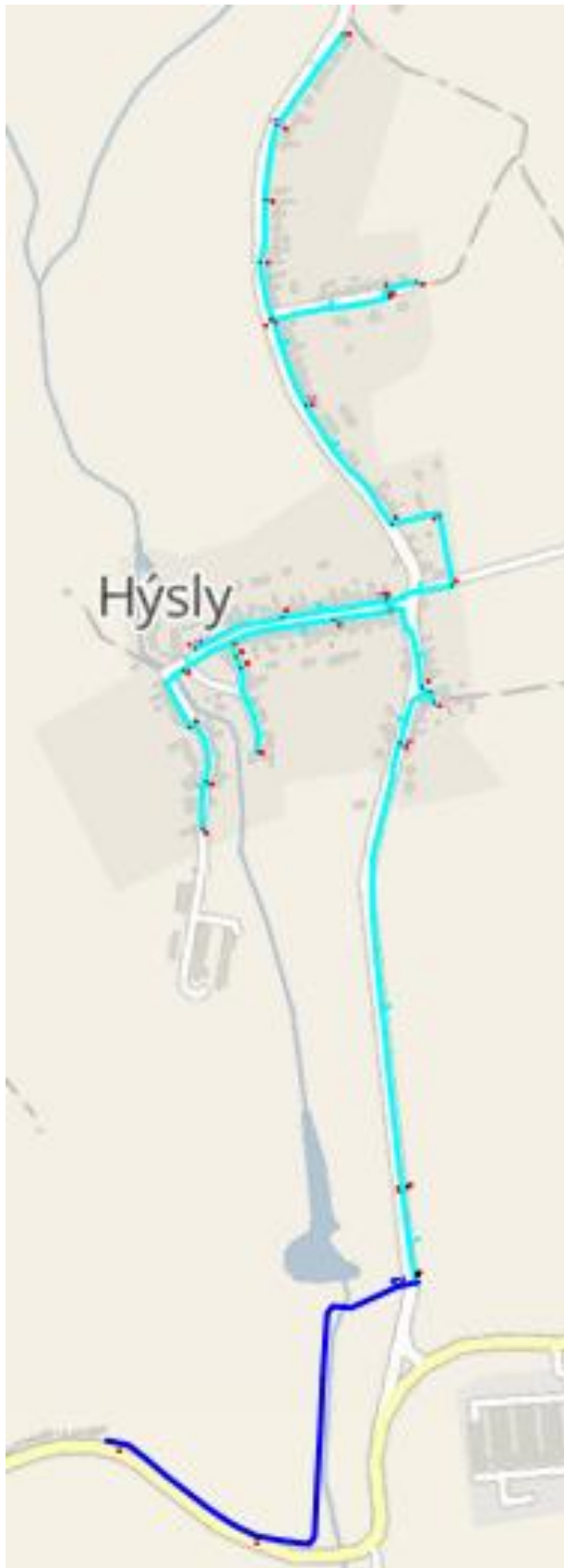
Obrázek č. 2: Vodovodní síť v obci
