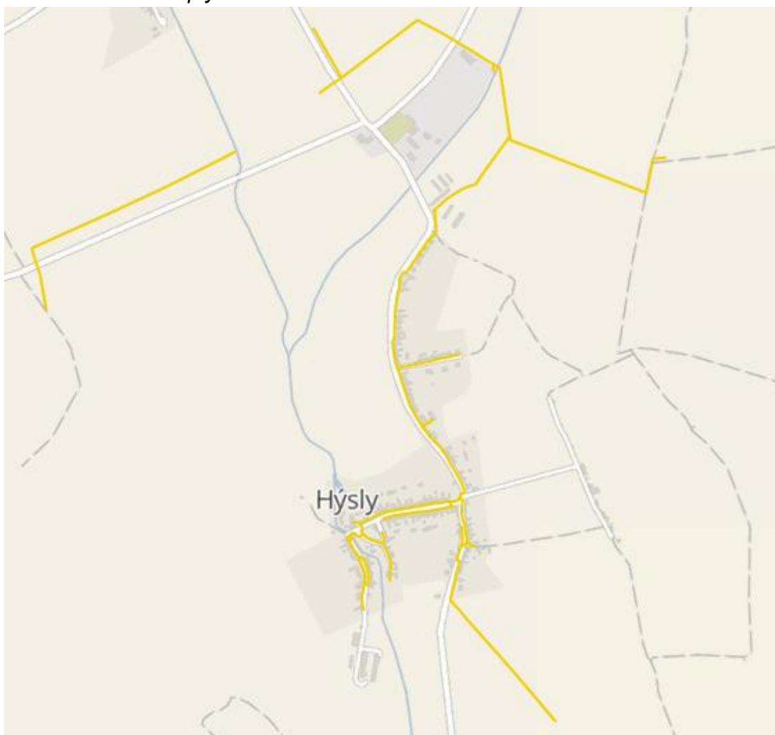
Obrázek č. 4: Vedení plynovodu v obci
