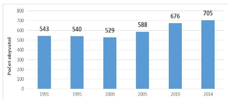
Graf č. 1 Vývoj počtu obyvatel obce Mokrovraty
