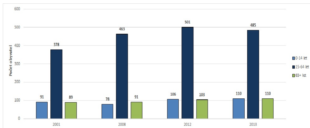
Graf č. 2 Vývoj jednotlivých věkových kategorií obyvatel obce
