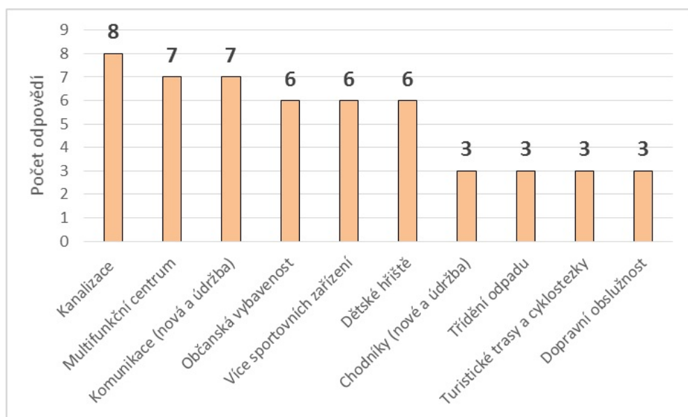
Graf 5 Co lidem v obci nejvíce chybí
